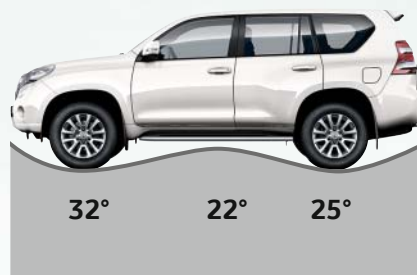
Vrijloophoek voor, overklimhoek en vrijloophoek achter
